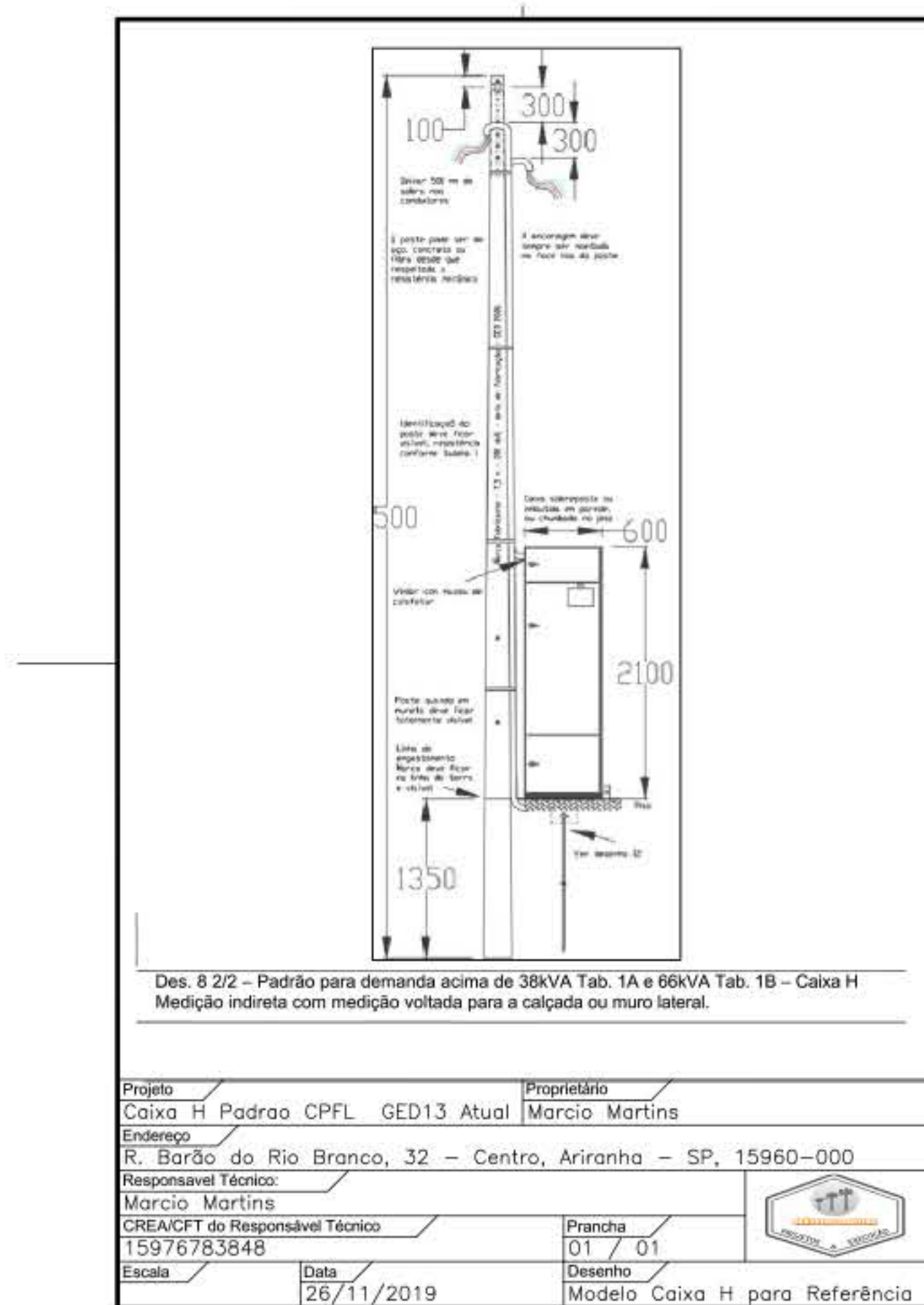
Projeto Caixa H Padrão CPFL
