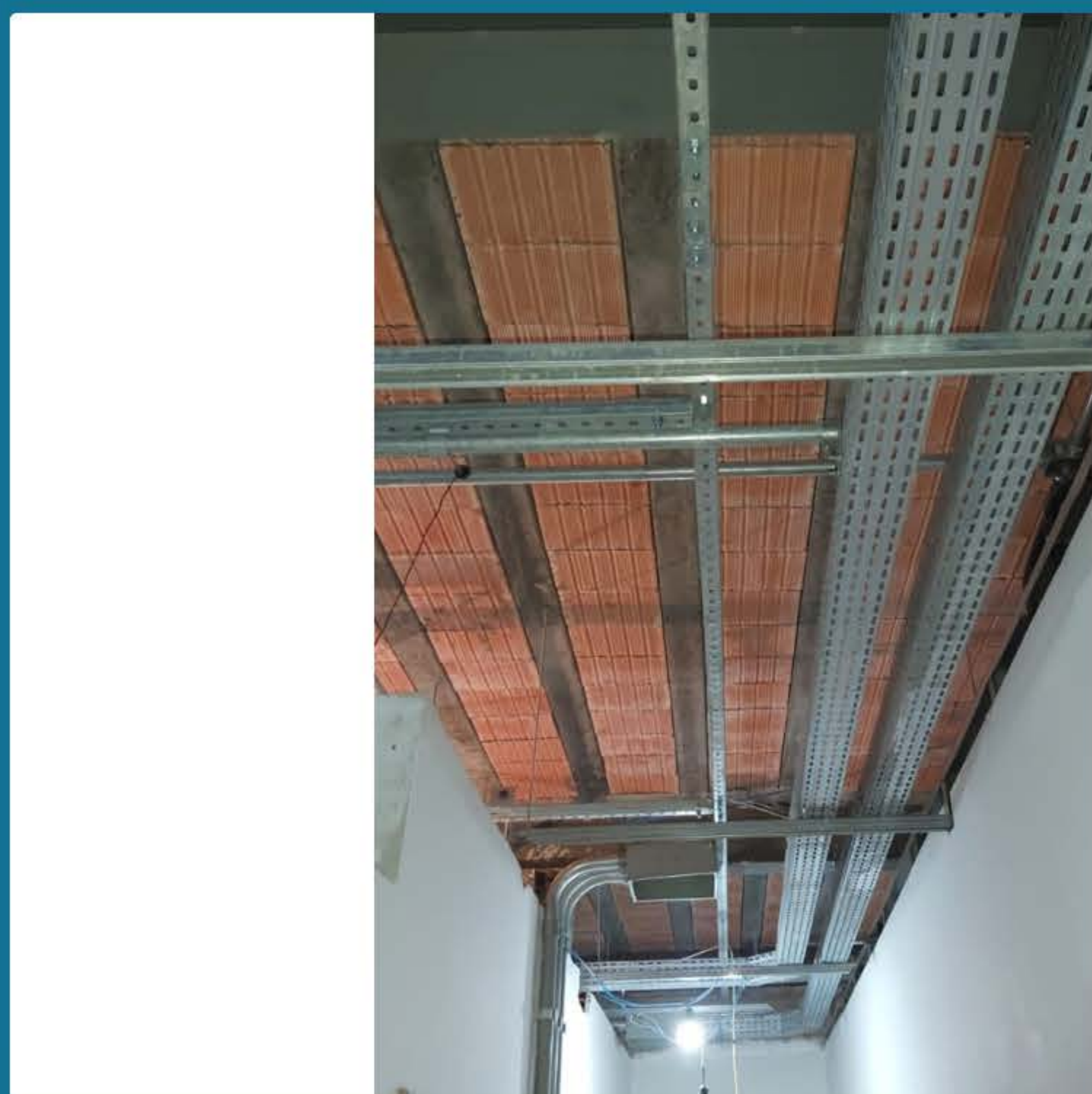
Obras de Infraestrutura
