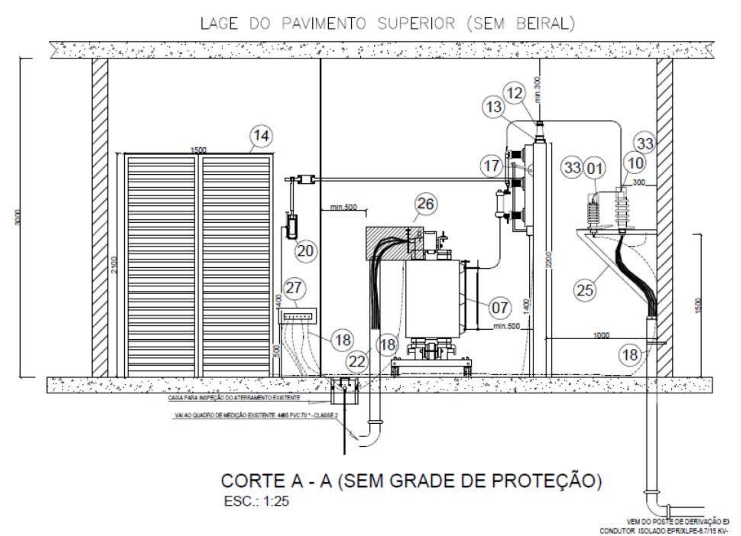
Projeto Subestação Abrigada
